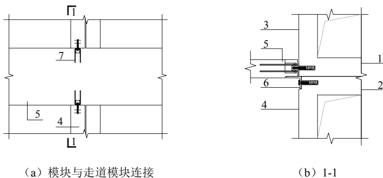
图 6.5.6 模块与走道模块连接示意图
