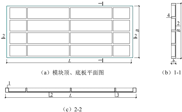
图 6.3.3-1 模块顶、底板构造示意图
