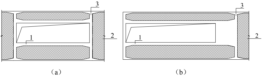
图 6.3.6-1 模块顶、底板开洞示意图
