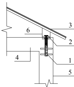
图 6.5.6 模块与屋架连接示意图
