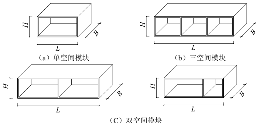
图 5.2.1 通用型模块
