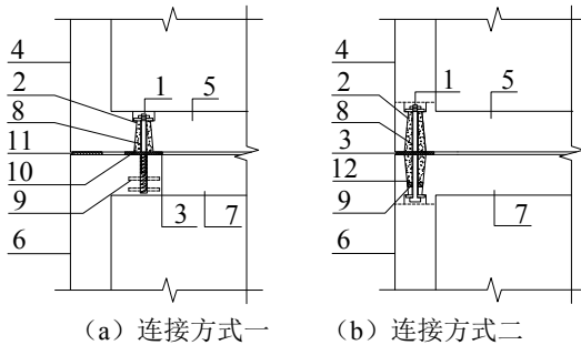
图 A.0.2 模块连接示意图
