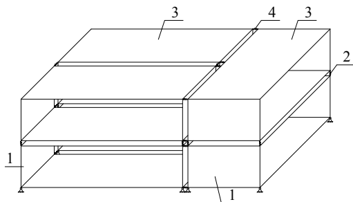
(b) 空间模型
