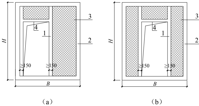
图 6.3.6-2 模块墙板开洞示意图
