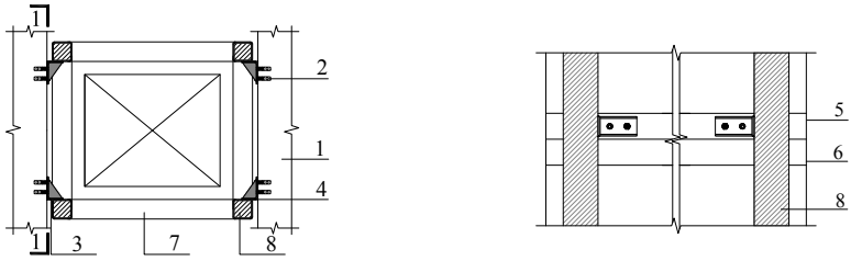
(a) 模块与钢结构电梯间连接示意图
