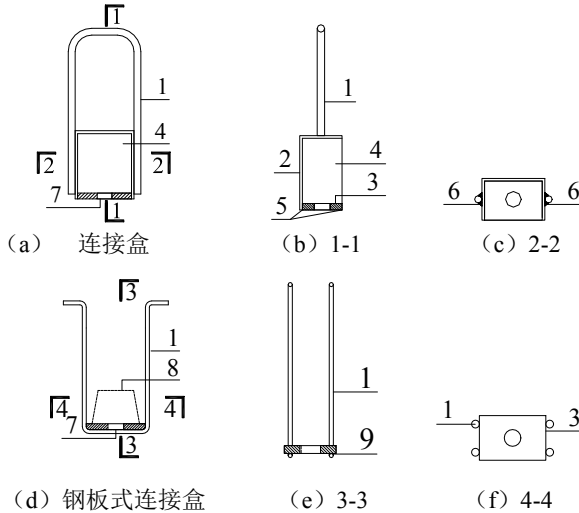
图 A.0.1 连接盒示意图
