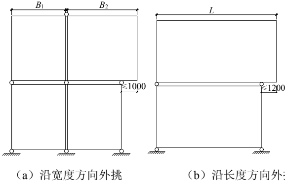
图 6.2.3 悬挑示意图
