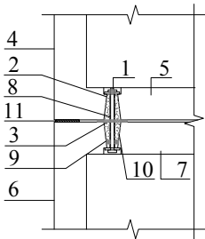
(a) 模块连接（边跨）
