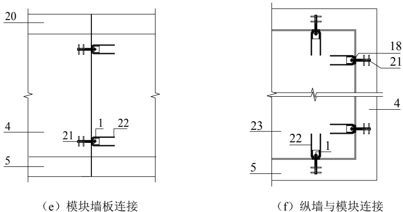
图 6.5.5-2 模块连接示意图
