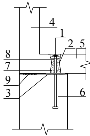
图 6.5.5-1 模块墙板与基础连接
