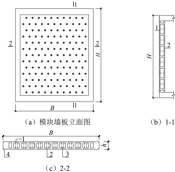
图 6.3.2-2 模块墙板构造示意图
