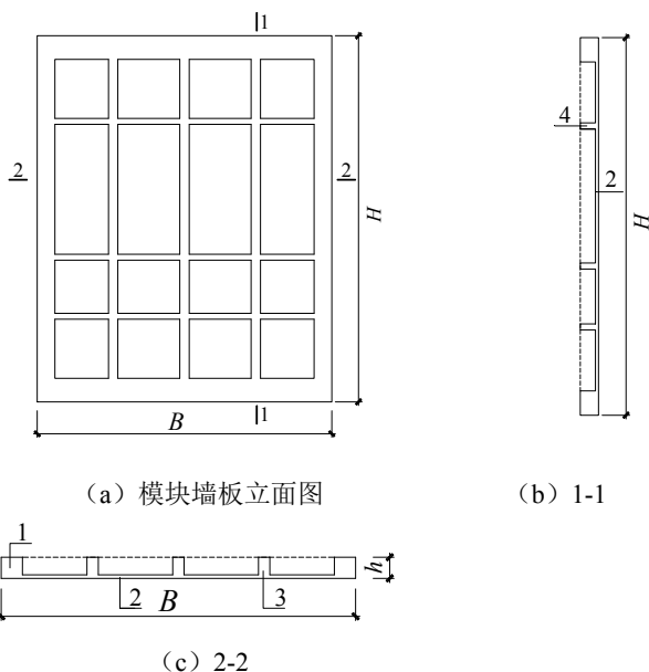
图 6.3.3-2 模块墙板构造示意图
