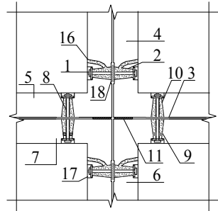
(b) 模块连接（中跨）
