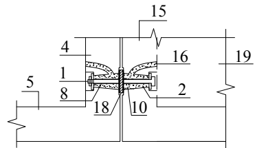
(d) 模块外侧墙与模块墙体纵横连接
