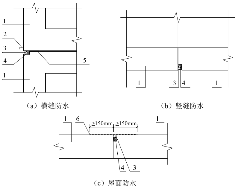
图 5.4.4 建筑防水示意
