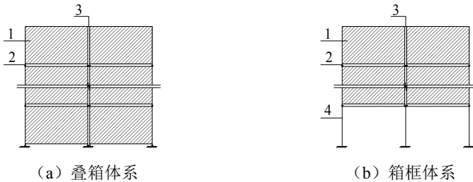
图 6.2.1 模块建筑结构体系示意图
