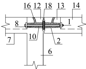
(c) 模块楼板纵横连接
