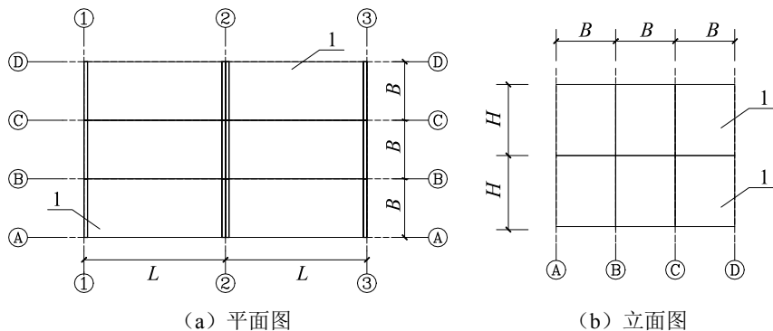
图 5.2.2 定位轴线示意图
